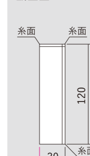
断面図
